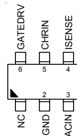
SOT-23-6
