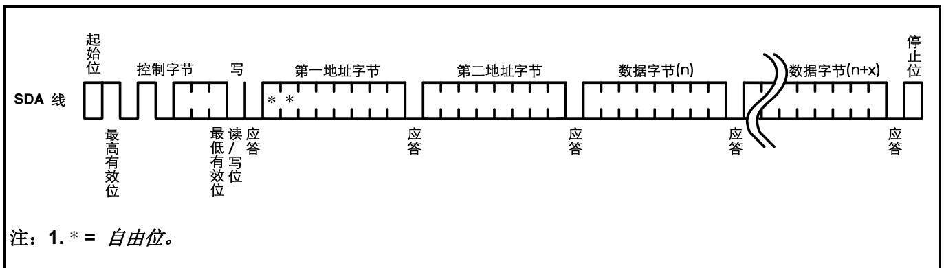
图 9. 页写
