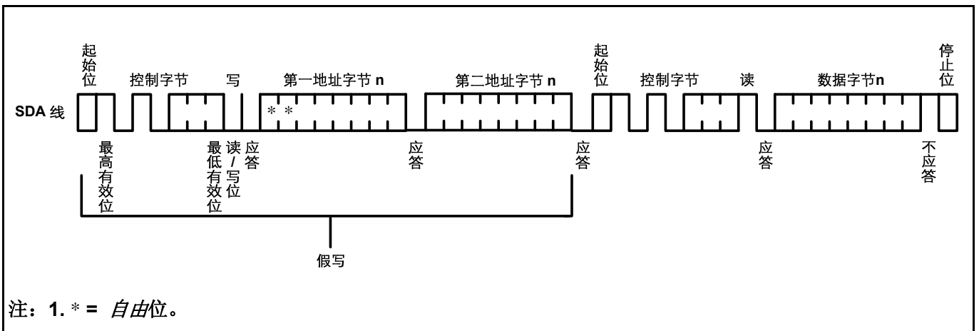
图 11. 自由读
