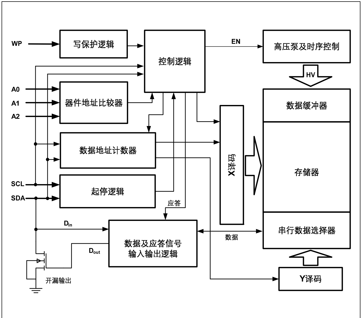
图 1. 结构框图
